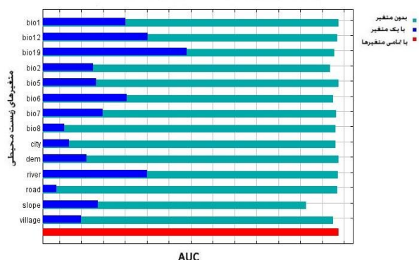
شکل ۵: نمودار آزمون جک نایف جهت بررسی میزان نقش هریک از متغیرها در اعتبار مدل
