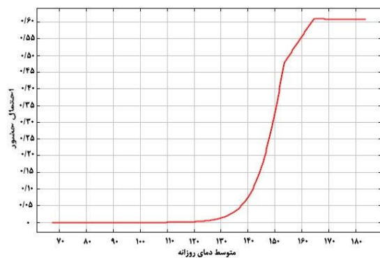
شکل ۸: منحنی پاسخ متوسط دمای روزانه
